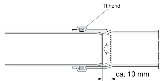
Joonis 24. Toruotsa ühendamine muhviga
